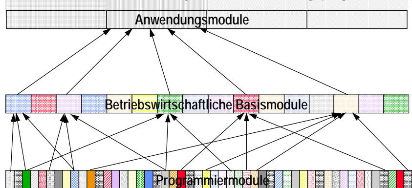
Vereinfachtes Schichtenmodell der Modularität
